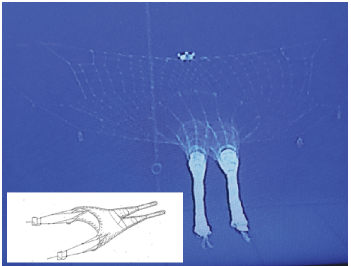
Общий вид пелагического двухмотенного трала
